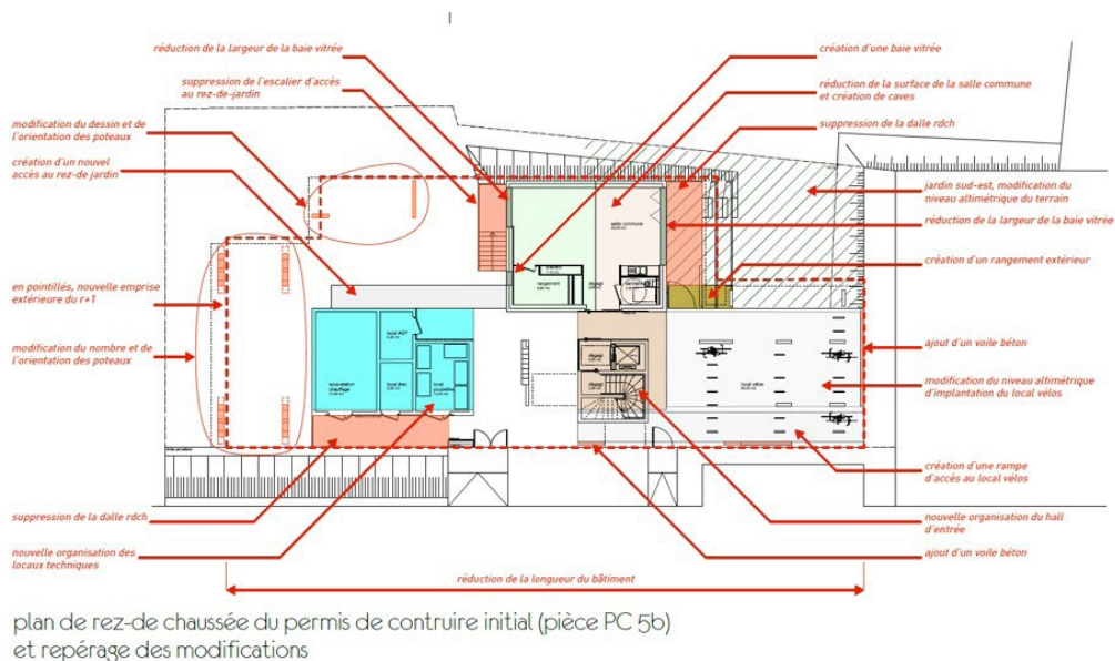
Illustration 3 : Plan qui illustre la réduction de moitié de la salle commune en cours de projet, plan de l'agence d'architecture
